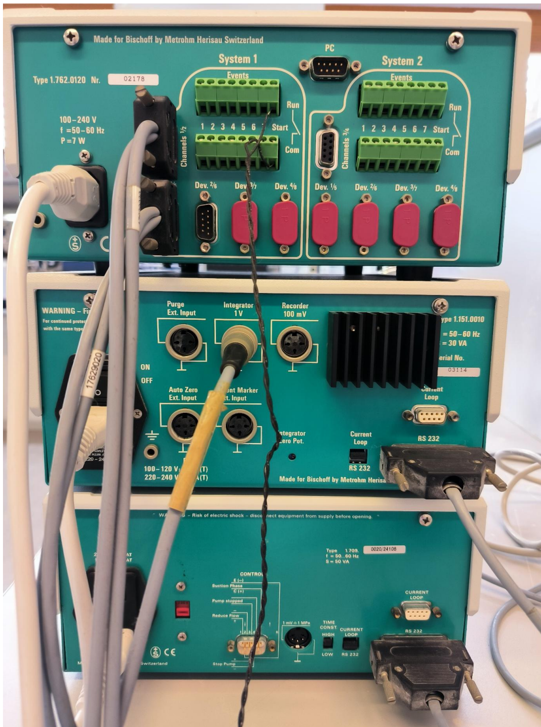
HPLC- Pumpe, RI-Detektor, Interface _hinten · Bild 2
